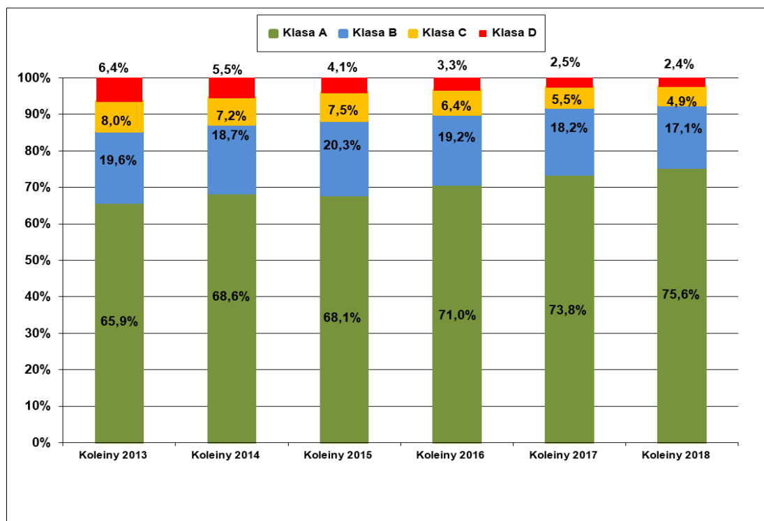
Rysunek 14. Zmiany równości poprzecznej (głębokości kolein)
