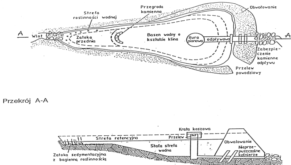
Rys. 2.7. Zbiornik retencyjny ze stałą strefą wodną wg [22]
