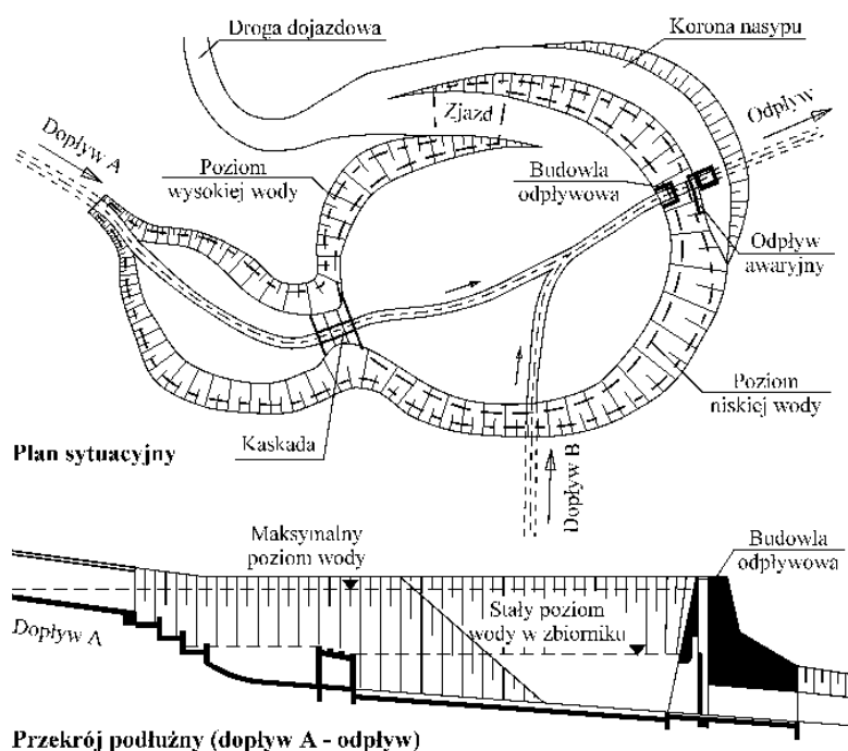
Rys. 2.4. Zbiornik retencyjny otwarty– przykład rozwiązania z dużą różnicą poziomów dopływu i odpływu wg [10]
