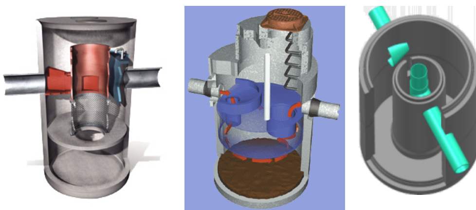
Rys. 2.19. Przykłady różnych rozwiązań osadników z przepływem wirowym [38]
