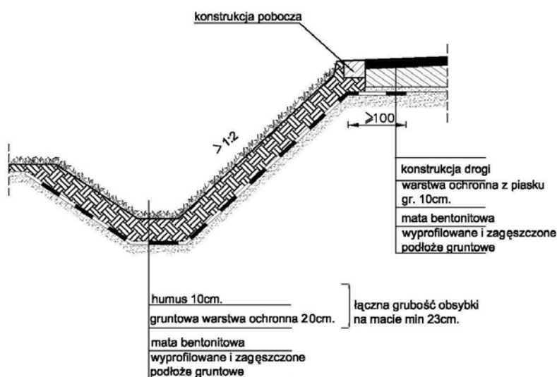
Rys. 2.14. Przykład uszczelnienia matą bentonitową rowu odwodnieniowego przy wysokiej skarpie drogowej - z kotwieniem poprzez wywiniecie na powierzchnię poziomą (nachylenie > 1:2 )
