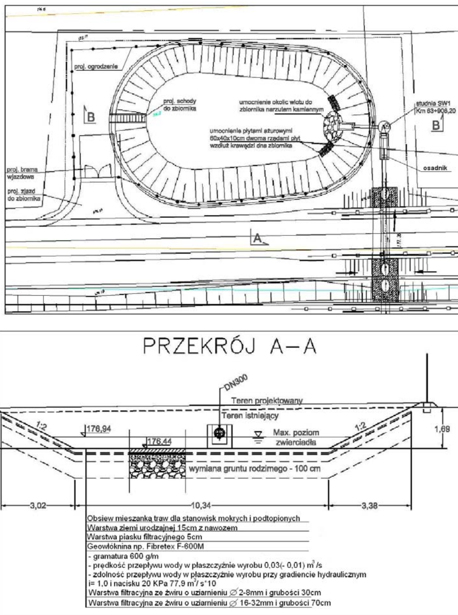
Rys. 2.3.B. Zbiornik infiltracyjny – przykład projektowy
