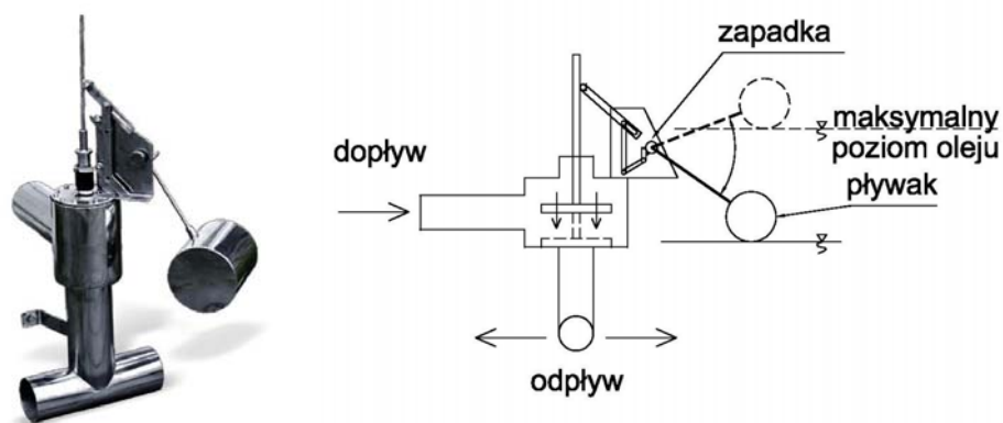
Rys. 2.25. Przykładowe rozwiązanie [41] i zasada działania śluzy dopływu
