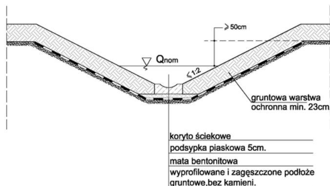
Rys. 2.13. Przykład uszczelnienia matą bentonitową rowu odwodnieniowego - bez konieczności dodatkowego kotwienia (nachylenie \leq 1:2 )
