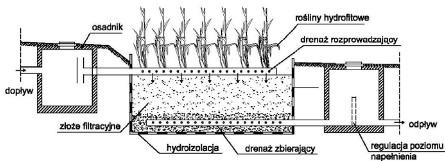
Rys. 2.10. Schematyczny przekrój filtra hydrofitowego o przepływie pionowym
