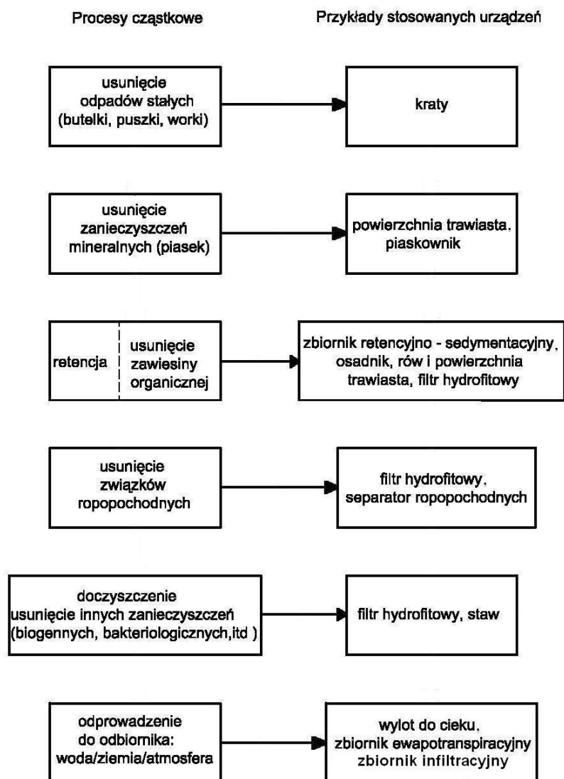
Rys. 2.11. Przykładowy schemat sposobów oczyszczania wód opadowych z pasa drogowego
