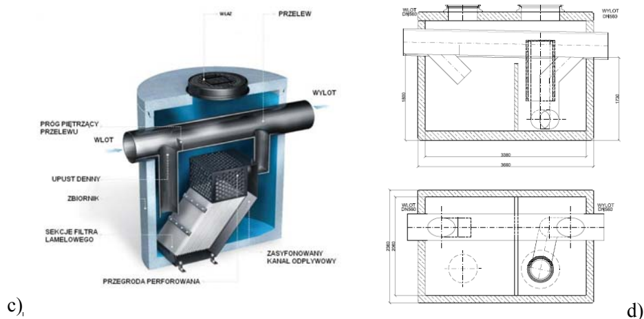
Rys. 2.22. Przykłady przelewów zintegrowanych [41]:
