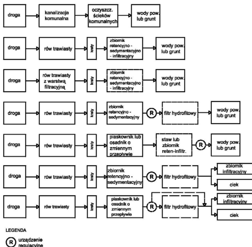
Rys. 3.3. Przykłady systemów oczyszczania ścieków opadowych z liniowych odcinków dróg i drogowych obiektów inżynierskich na terenach średnio wrażliwych
