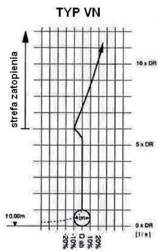
Rys. 2.29. Przykładowa charakterystyka hydrauliczna regulatora z kryzą dławiącą
