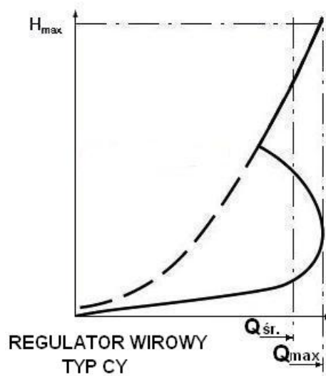
Rys. 2.30. Przykładowa charakterystyka hydrauliczna regulatora wirowego
