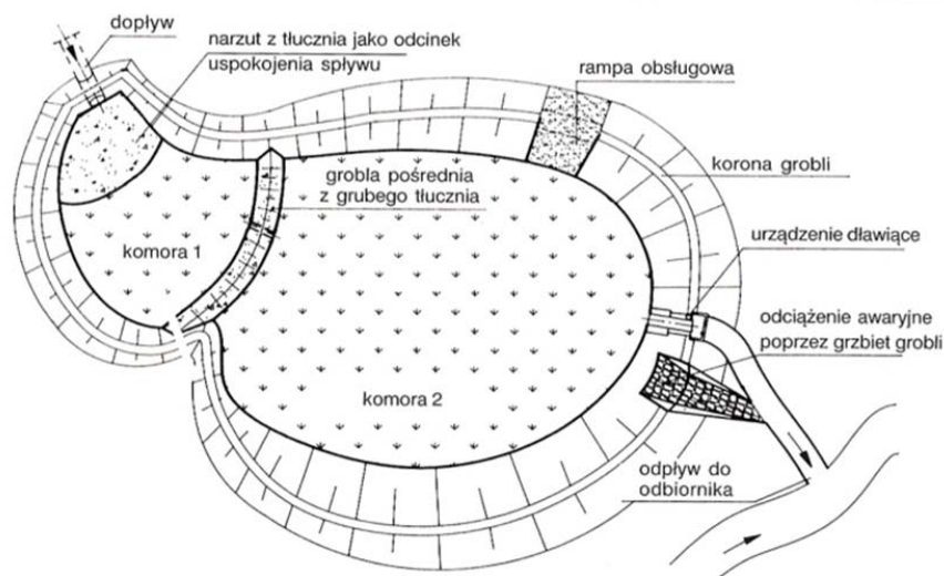
Rys. 2.5. Schemat ideowy stawu retencyjnego [13]
